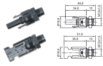
板端连接器 Panel Receptacle
